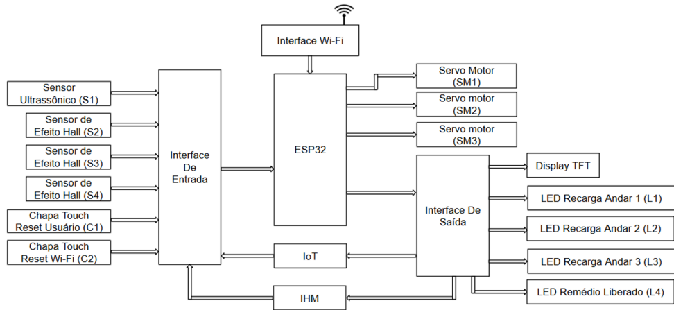
Diagrama de Blocos ESP32 – Modelo Completo
