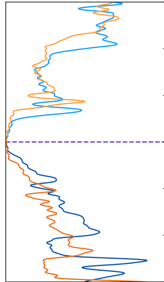
DOS (a.u.)
