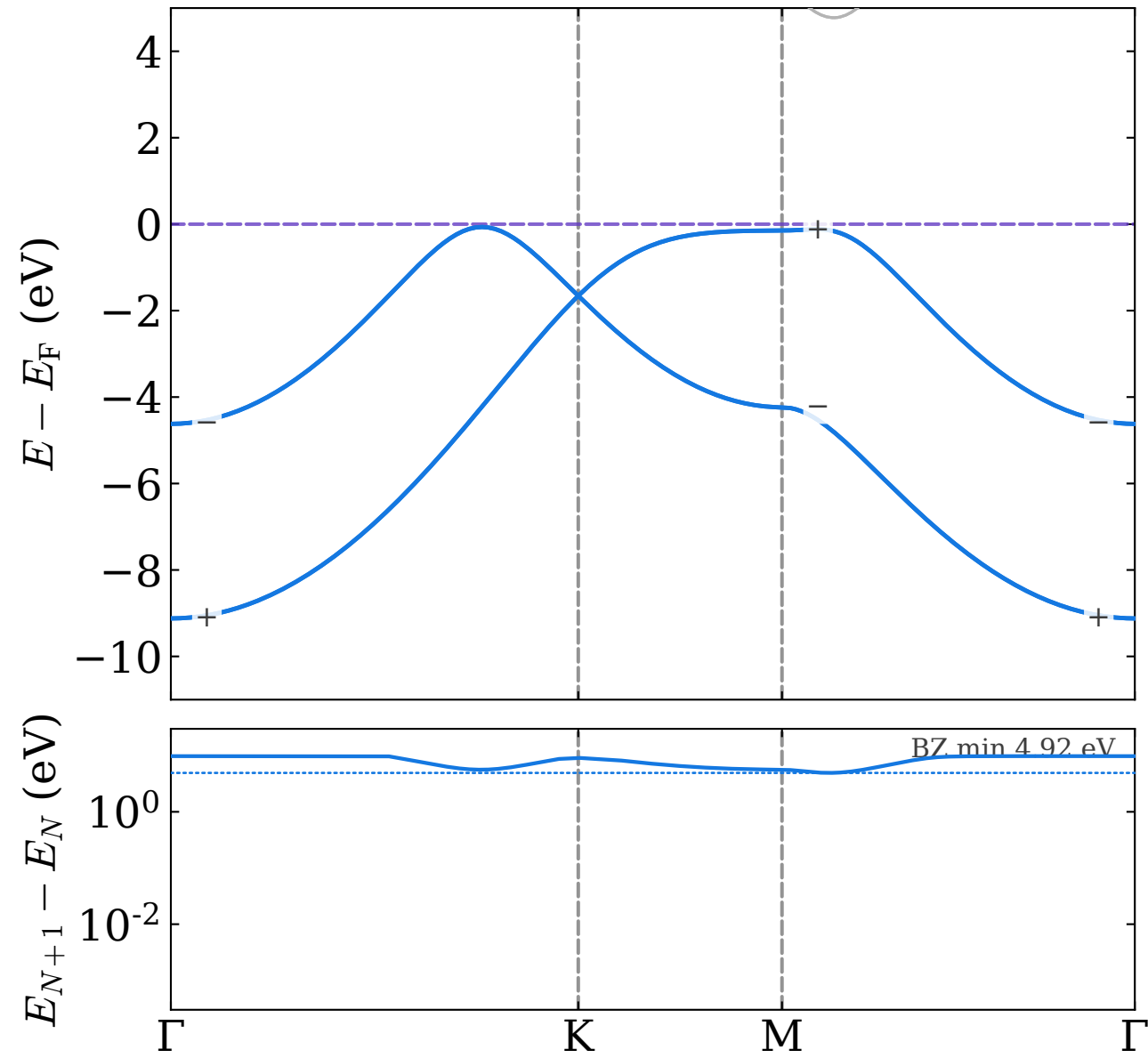
2H- \alpha -beryllene: \nu = 0
