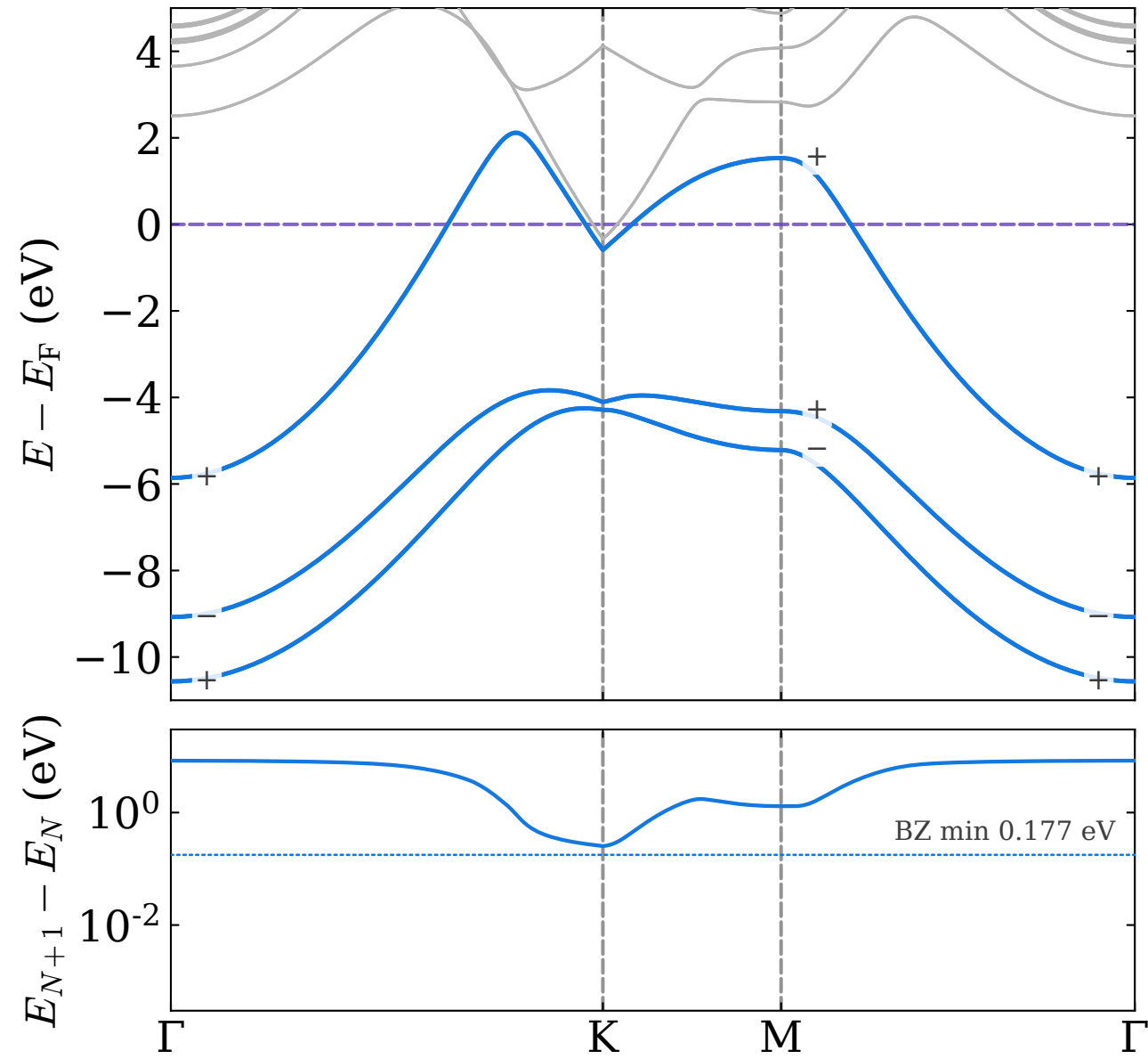
2H- \beta -beryllene: \nu = 0
