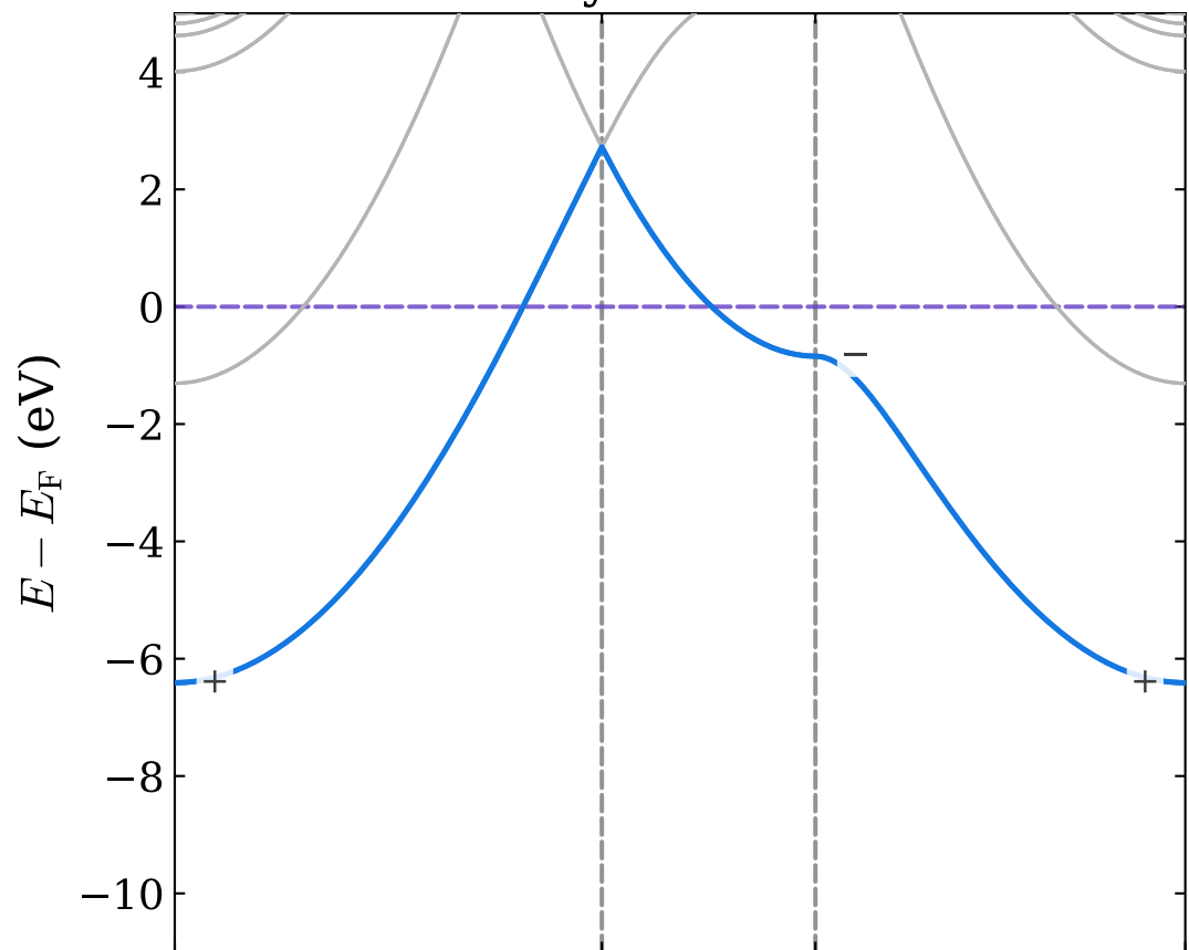
\alpha -beryllene: \nu = 1
