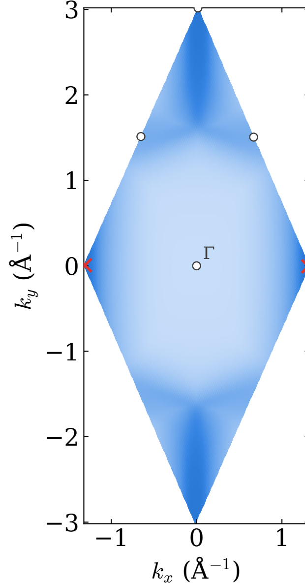
2H- \beta -beryllene, N = 6 min 0.177 eV
