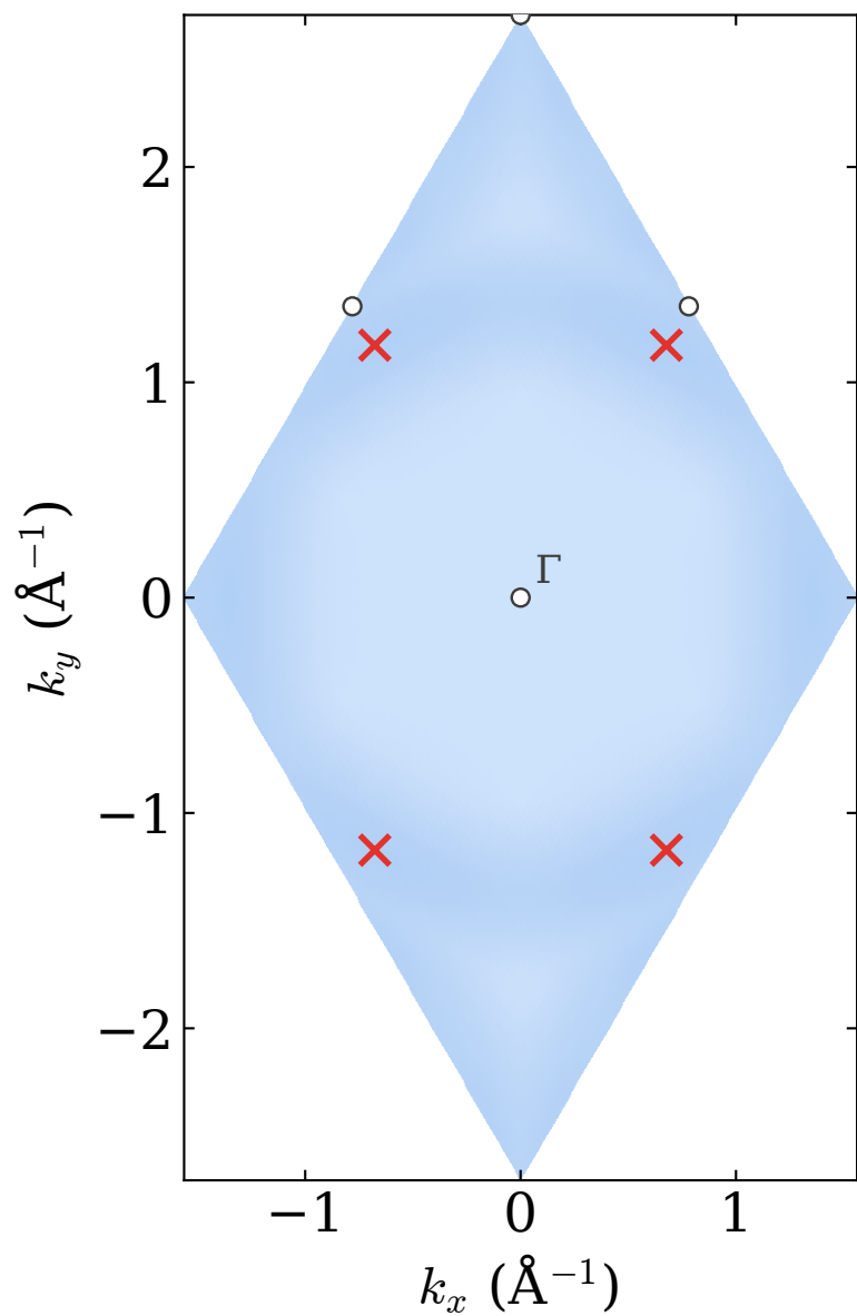
2H- \alpha -beryllene, N = 4 min 4.92 eV
