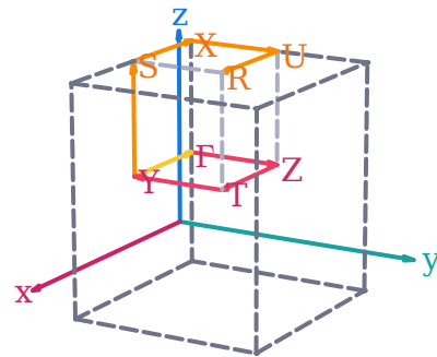
(b) Brillouin zone
