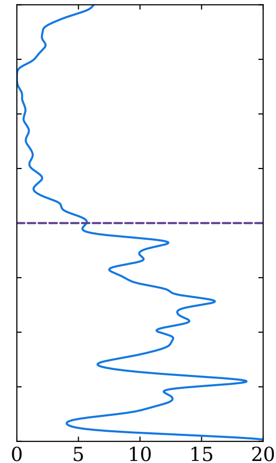
DoS (a.u.)
