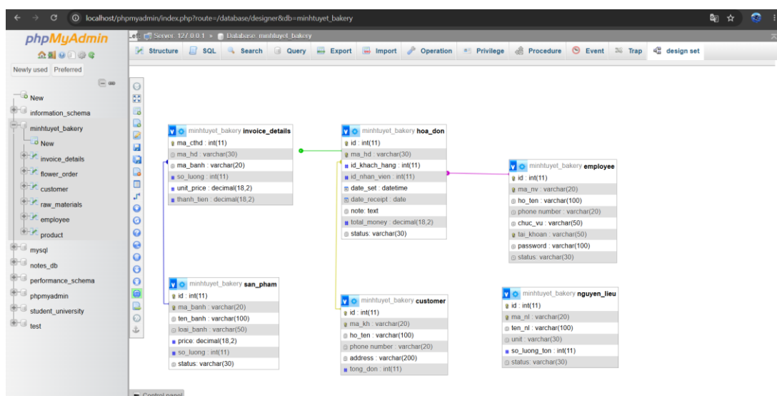
Hình 3.1 Sơ đồ CSDL ERD
