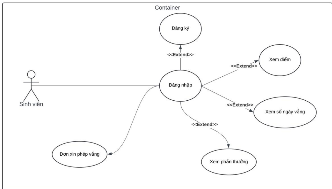
Hình 8: Sơ đồ Use case Sinh viên
