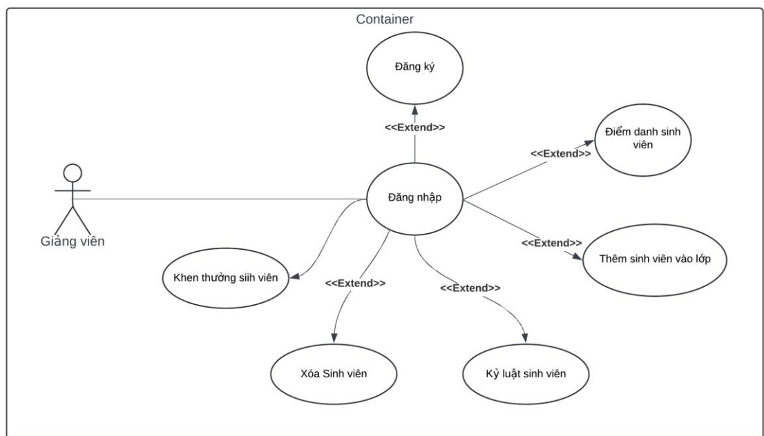
Hình 9: Sơ đồ Use case Giảng viên
