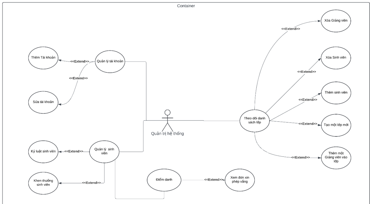
Hình 7: Sơ đồ Use case Quản trị hệ thống
