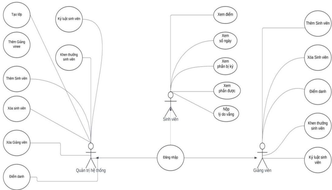
Hình 6: Sơ đồ Use case tổng thể
