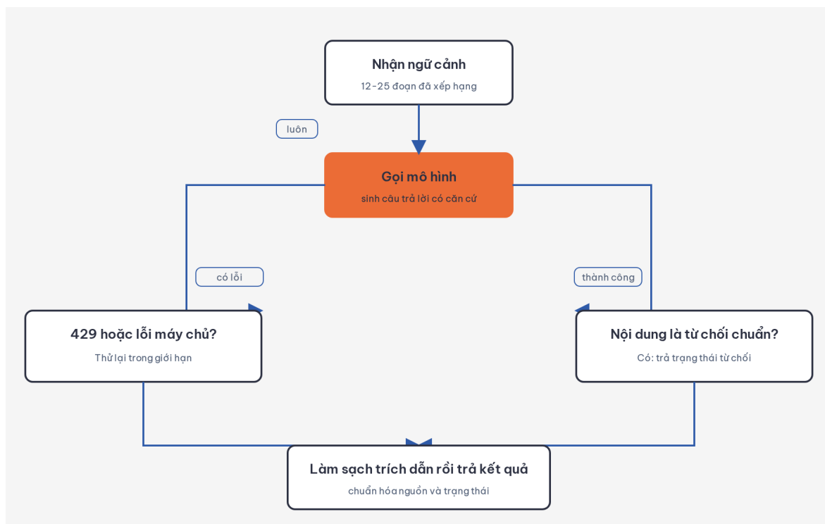
Hình 2.12: Bộ sinh câu trả lời trả lời một phần dựa trên ngữ cảnh đã truy xuất và bổ sung
