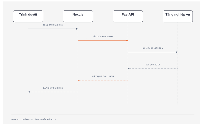
Hình 2.17: Vòng đời một yêu cầu HTTP giữa trình duyệt và FastAPI
