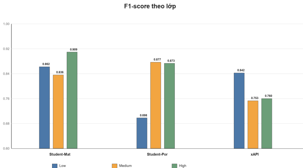
Hình 5.4. F1-score theo từng lớp Low, Medium và High Nguồn: Tác giả tổng hợp từ kết quả thực nghiệm của hệ thống.
