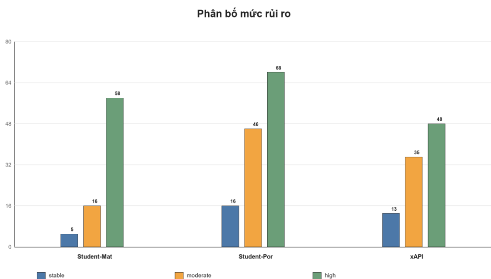
Hình 4.7. Phân bố risk band do bộ luật sinh ra
