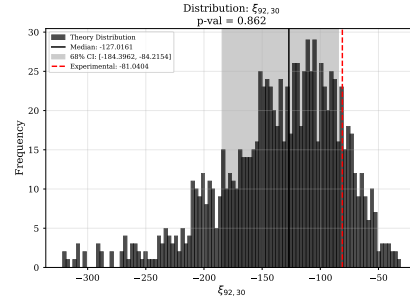
(d) \langle \xi \rangle_{30}^{92}
