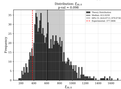
(e) \langle \xi \rangle_0^{30}
