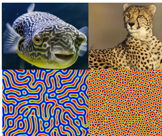
Figure 3.1.: Esempi di pattern di Turing in natura
