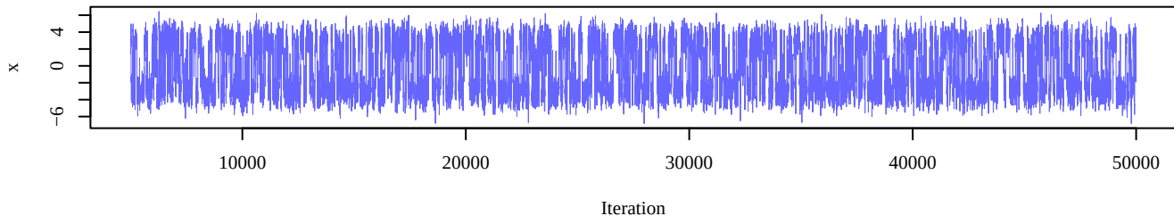
Posterior samples
