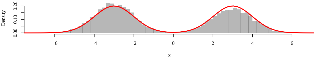
Posterior samples
