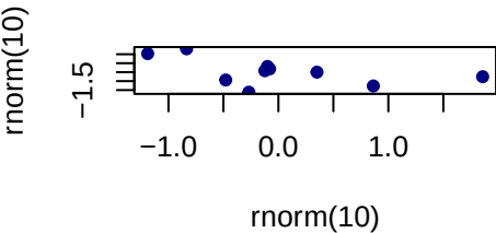
Scatter
