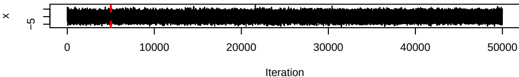
Posterior Samples (post burn-in)
