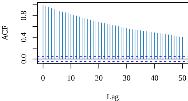
RW-MH Autocorr
