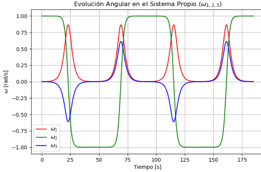
Figura 1: Evolución temporal de las componentes de la velocidad angular en el sistema de referencia solidario al cuerpo. La condición inicial corresponde a una rotación casi pura alrededor del eje intermedio, perturbada levemente en la dirección del eje 1.
