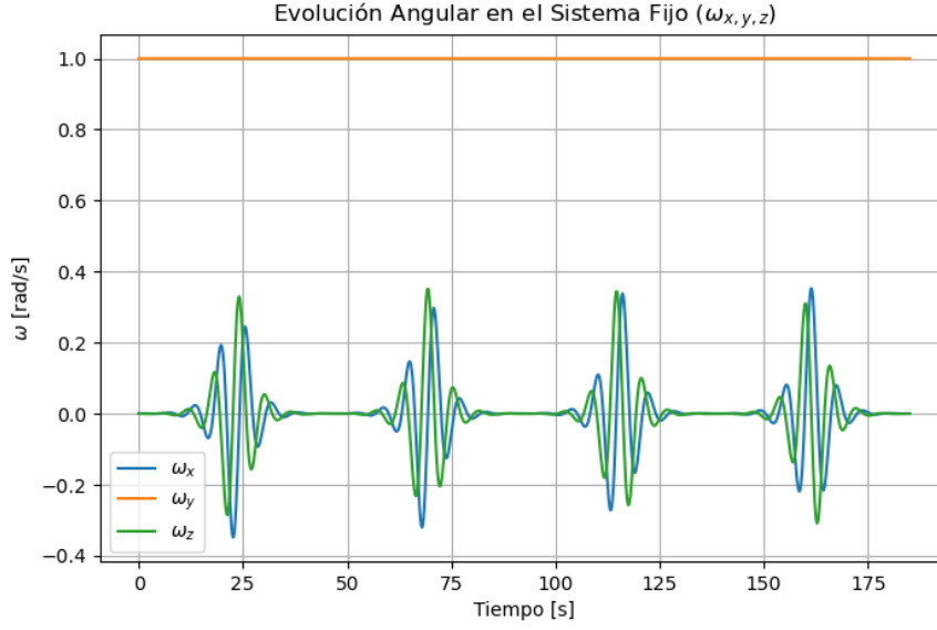
Figura 2: Componentes de la velocidad angular expresadas en el sistema inercial. La señal refleja la evolución de la actitud rotacional del cuerpo observada desde el laboratorio.
