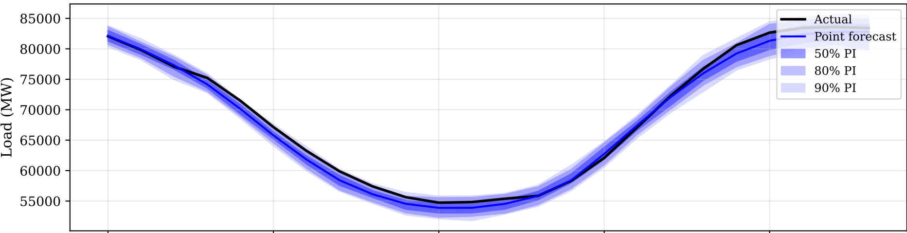
Moirai-2
