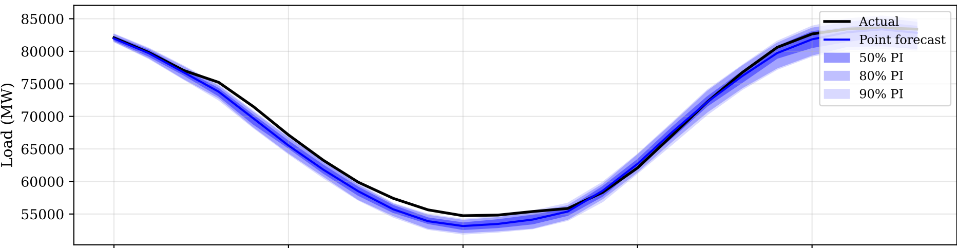
TTM
