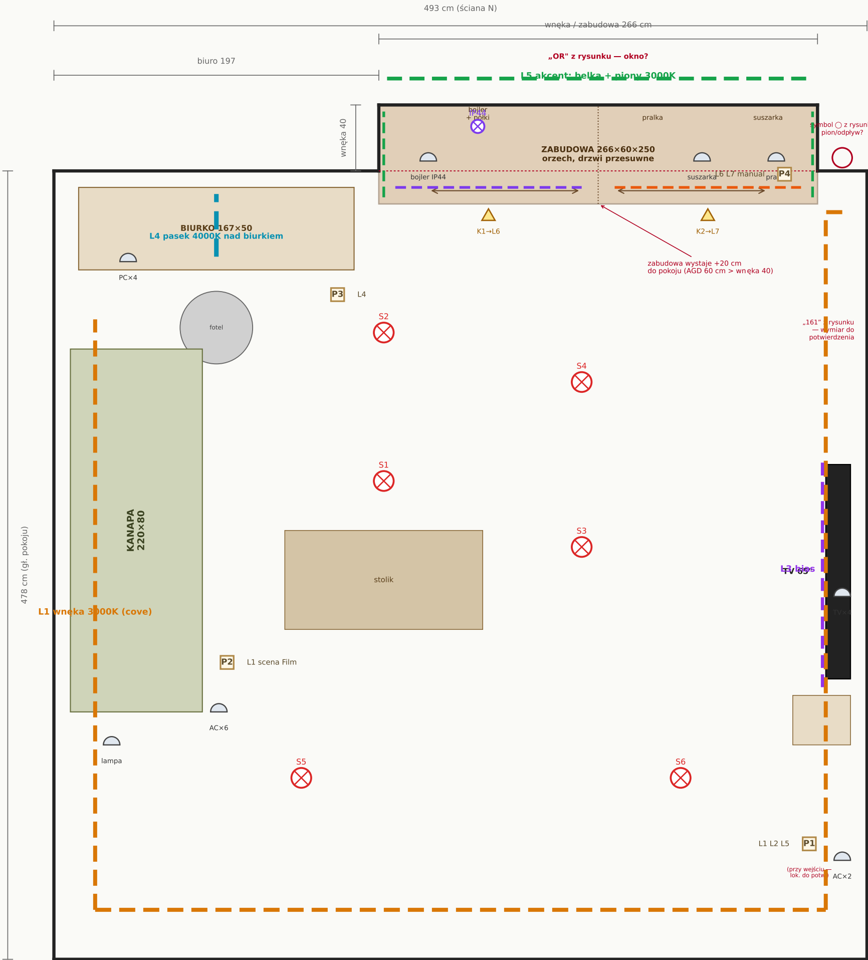
KARTA 1 / 3 · RZUT POMIESZCZENIA Z OŚWIETLeniem (v2, skorygowany) · 1:50
