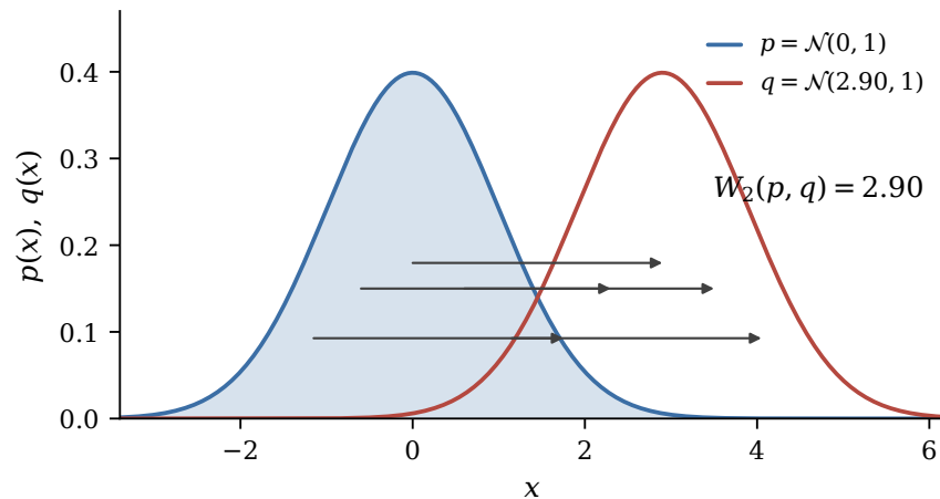
Wasserstein: long transport
