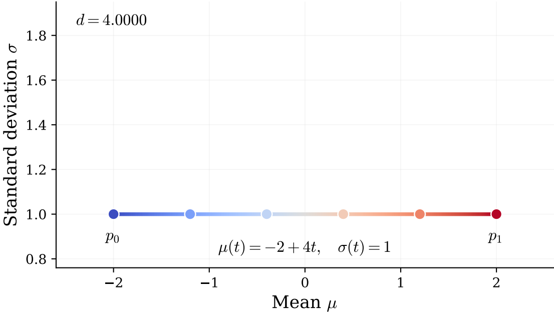
Wasserstein-Otto
