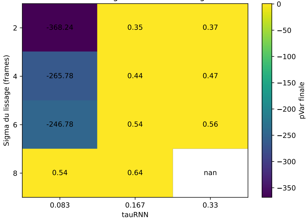
Souris 409 : grille tauRNN \times lissage
