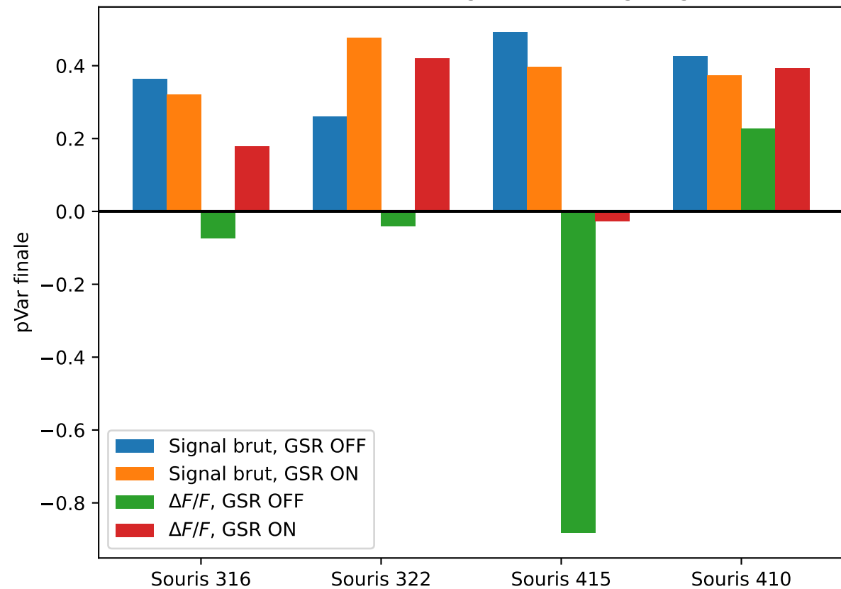
Effet du \Delta F/F et de la régression du signal global
