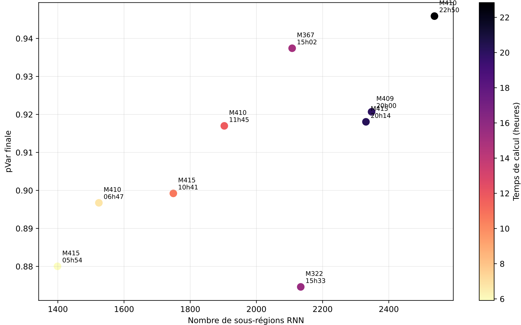
nRunTrain=100 : nombre de sous-régions vs pVar
