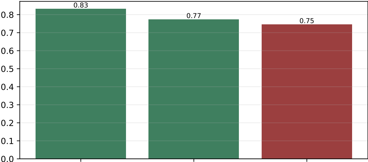
Correlation mediane des derivees
