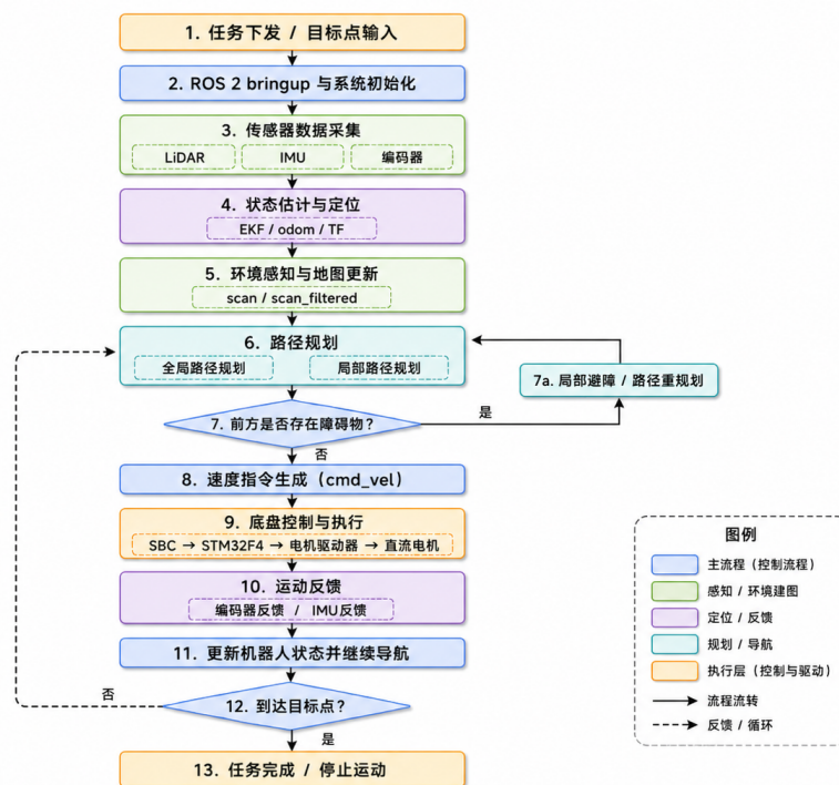
图 8.1: ROSbot XL 自主导航与底盘闭环控制流程图
