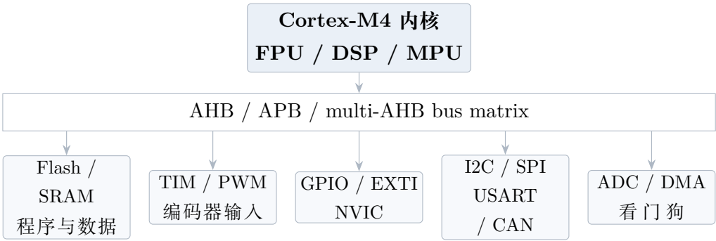
图 5.2: STM32F4 微控制器内部结构抽象图
