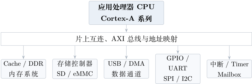
图 5.1: SBC 上位计算平台内部结构抽象图
