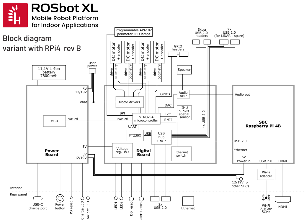
图 4.1: ROSbot XL 硬件系统框图
