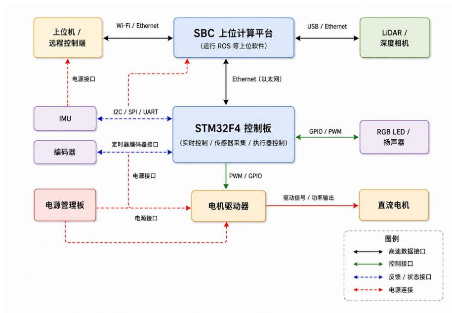
图 6.1: ROSbot XL 系统接口关系图
