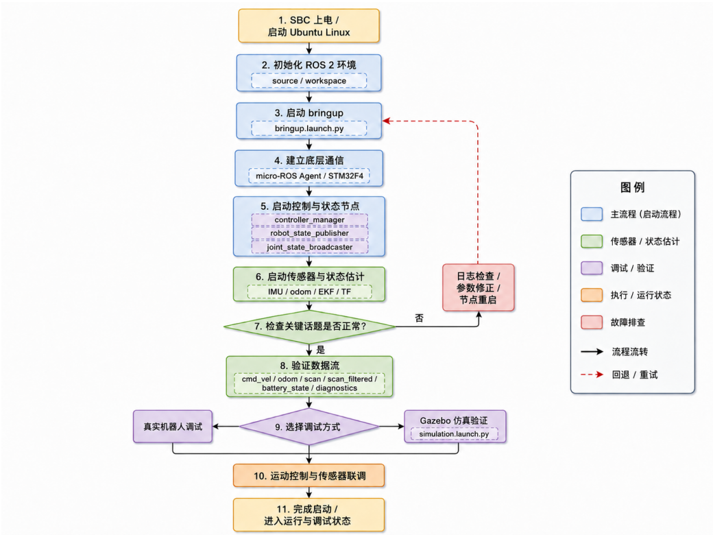
图 8.2: ROS 2 启动与调试流程图
