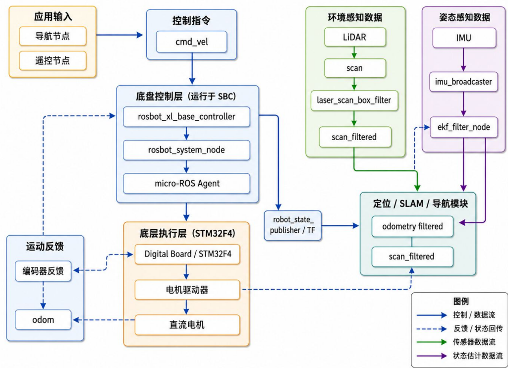
图 7.2: ROSbot XL ROS 2 软件数据流图
