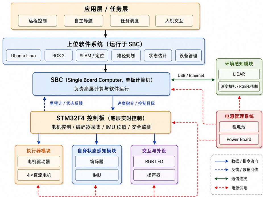
图 3.1: ROSbot XL 软硬件协同总体架构图
