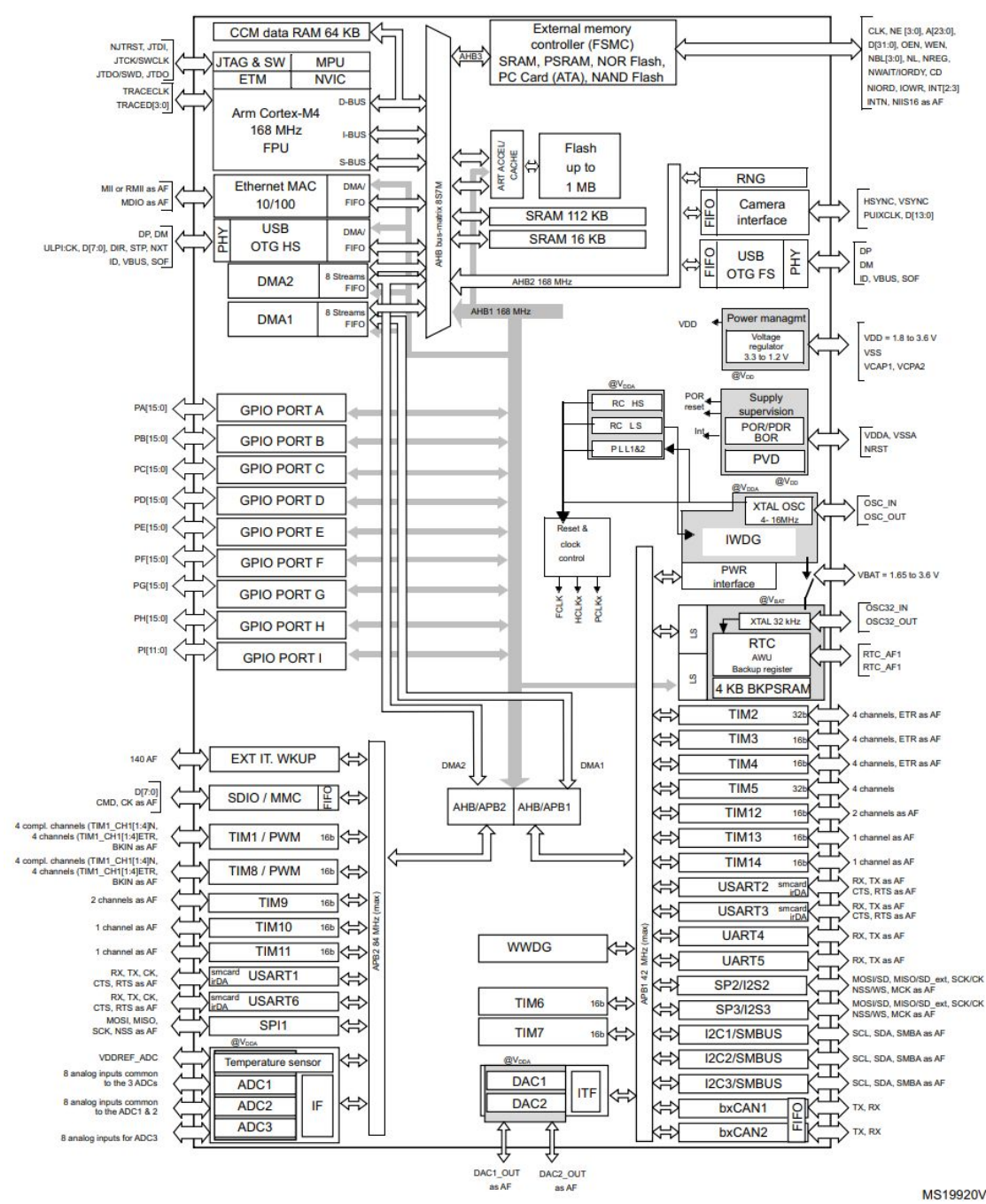
图 5.3: STM32F4 微控制器内部结构参考图
