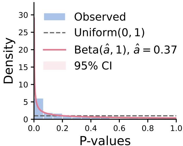
LMR P-Values
