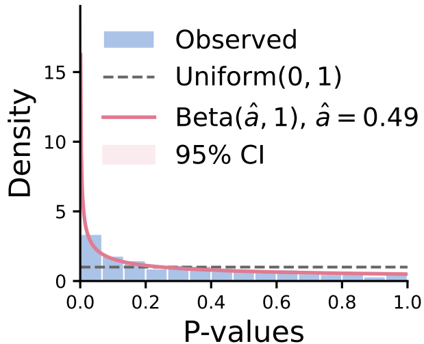
LMR P-Values
