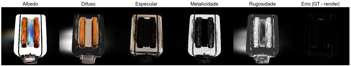
Figura 7. Mapas intermediários da renderização diferida na cena toaster (iteração 50.000, vista de treino): albedo, componentes difusa e especular, metalicidade, rugosidade e erro absoluto em relação à imagem real.
