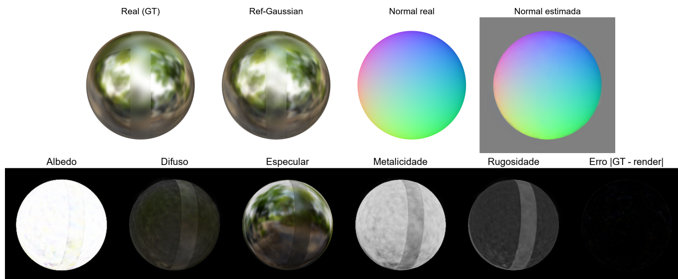
Figura 6. Cena ball , convexa e sem inter-reflexões. Acima: imagem real, renderização, normal real e normal estimada (vista de teste 0). Abaixo: mapas intermediários da renderização diferida (vista de treino). A faixa mais rugosa da esfera aparece clara na rugosidade e mais escura na metalicidade.
