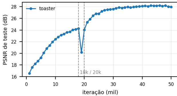
Figura 3. PSNR nas vistas de teste ao longo do treino da cena toaster (a ball foi treinada sem registro do log). As linhas tracejadas marcam o fim do sombreamento por Gaussiana (18 mil iterações) e o início da inter-reflexão (20 mil).
