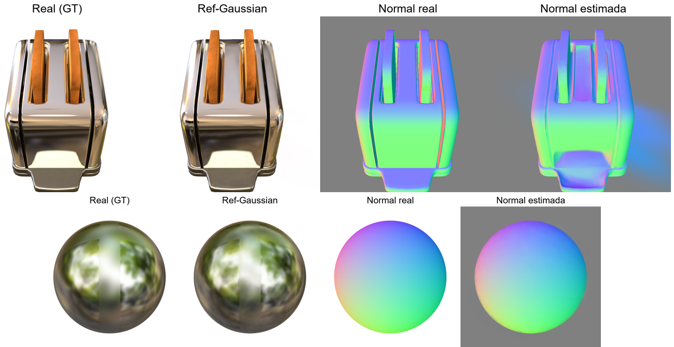
Figura 2. Resultados nas cenas toaster (acima) e ball (abaixo), na primeira imagem de teste. Da esquerda para a direita: imagem real, imagem gerada pelo Ref-Gaussian, normal real e normal estimada (as cores codificam a direção da superfície).
