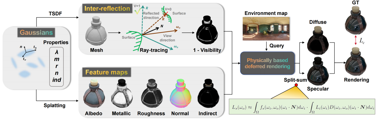
Figura 1. Visão geral do Ref-Gaussian. As Gaussianas guardam propriedades de material, que são projetadas em mapas por pixel; a cor final é calculada a partir desses mapas, da luz do ambiente e dos reflexos entre partes do objeto. Fonte: Yao et al. [3].
