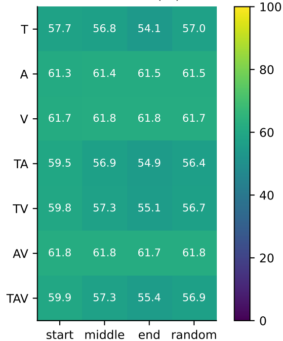
F Macro-F1 (%)
