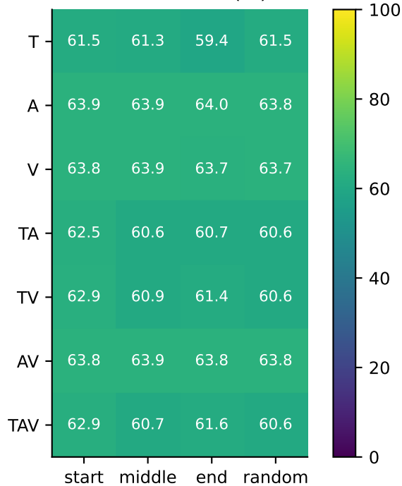
Bm Macro-F1 (%)
