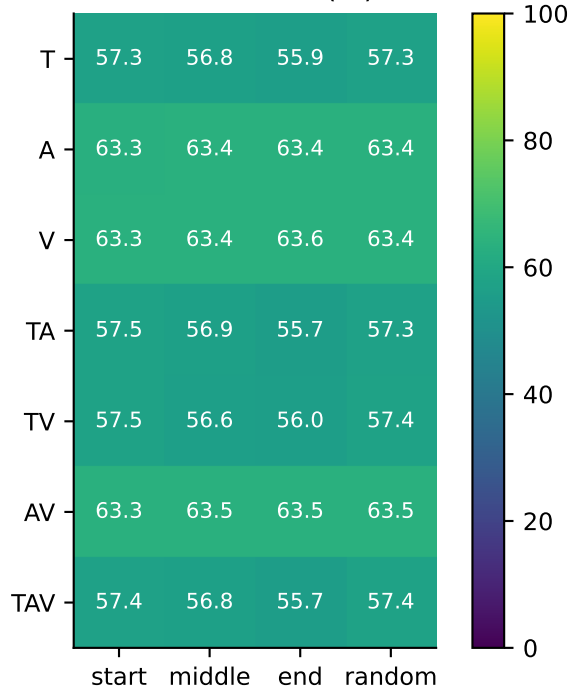
B0 Macro-F1 (%)
