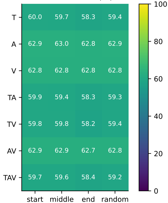
noC Macro-F1 (%)
