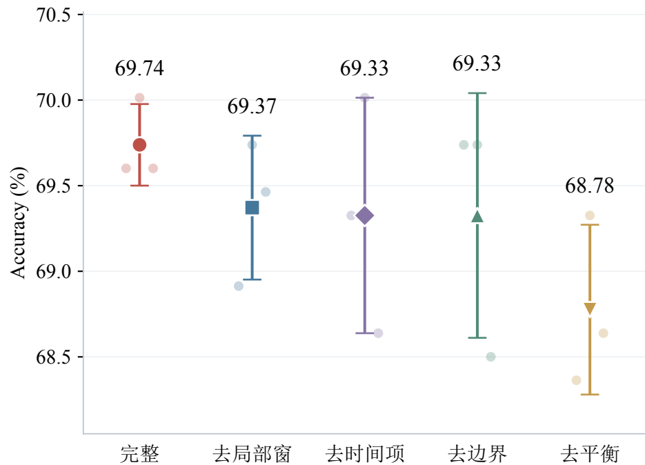
(e) 准确率
