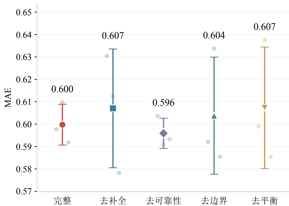
(c) 平均绝对误差
