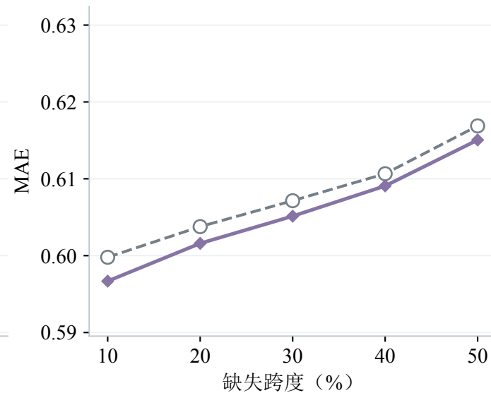
(c) 无可靠性
