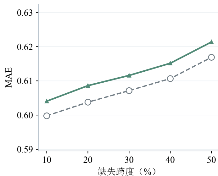
(d) 无边界损失
