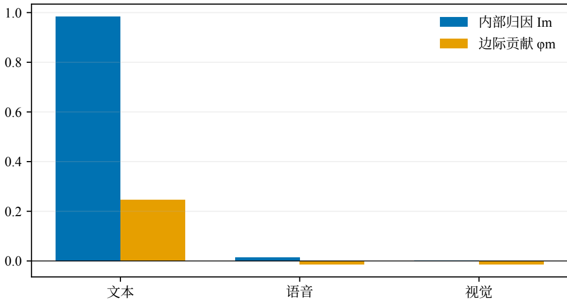
样本 01 三模态作用差异
