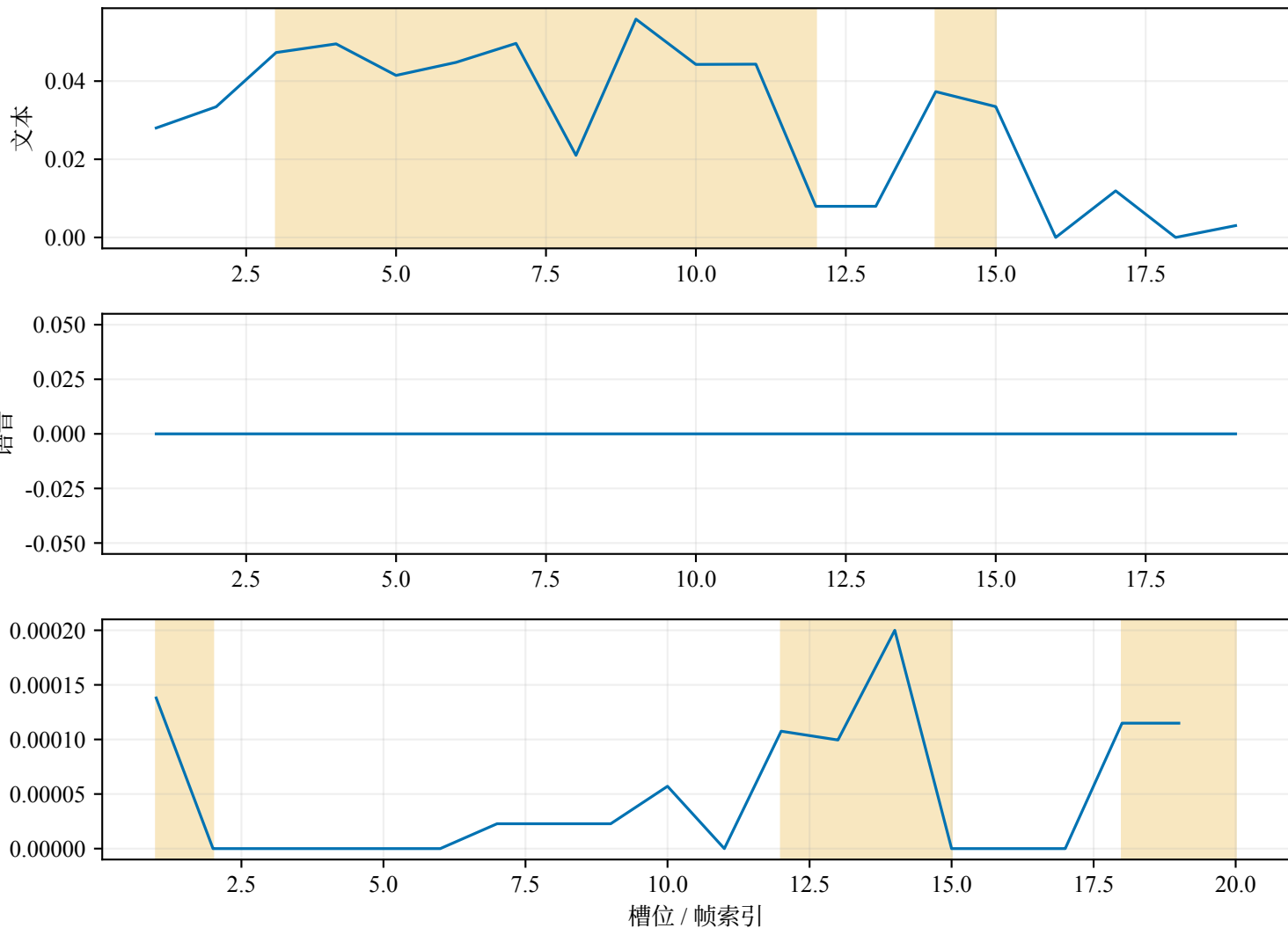
样本 02 正向 Grad×Input (阴影=支持当前预测的关键证据)
