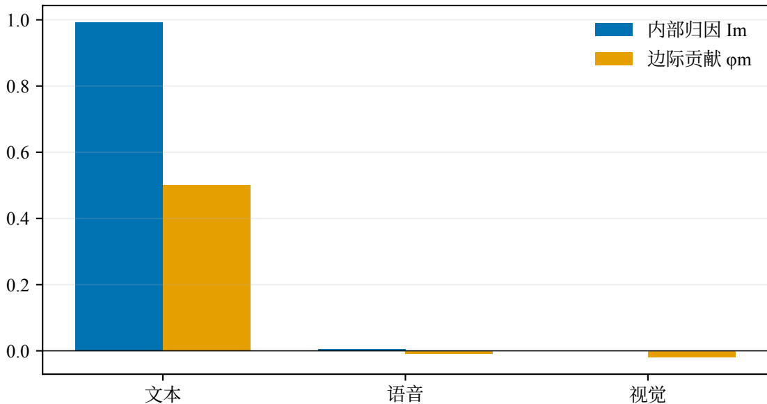
样本 04 三模态作用差异
