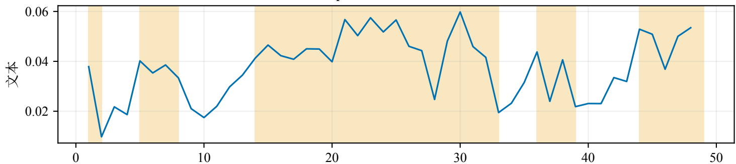
样本 07 正向 Grad×Input (阴影=支持当前预测的关键证据)
