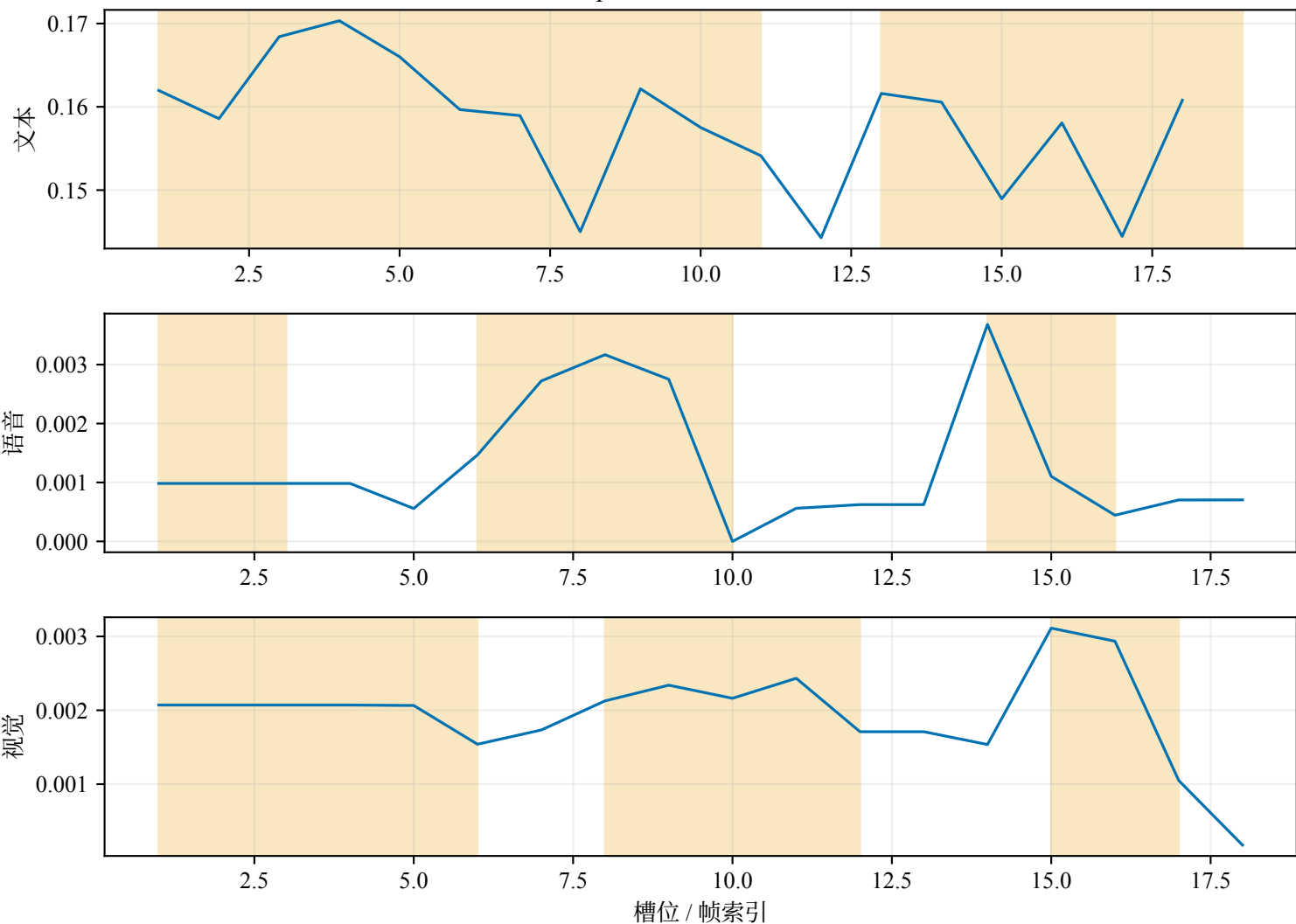
样本 09 正向 Grad×Input (阴影=支持当前预测的关键证据)
