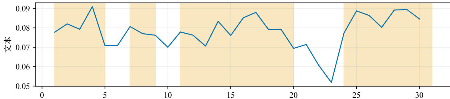
样本 10 正向 Grad×Input (阴影=支持当前预测的关键证据)
