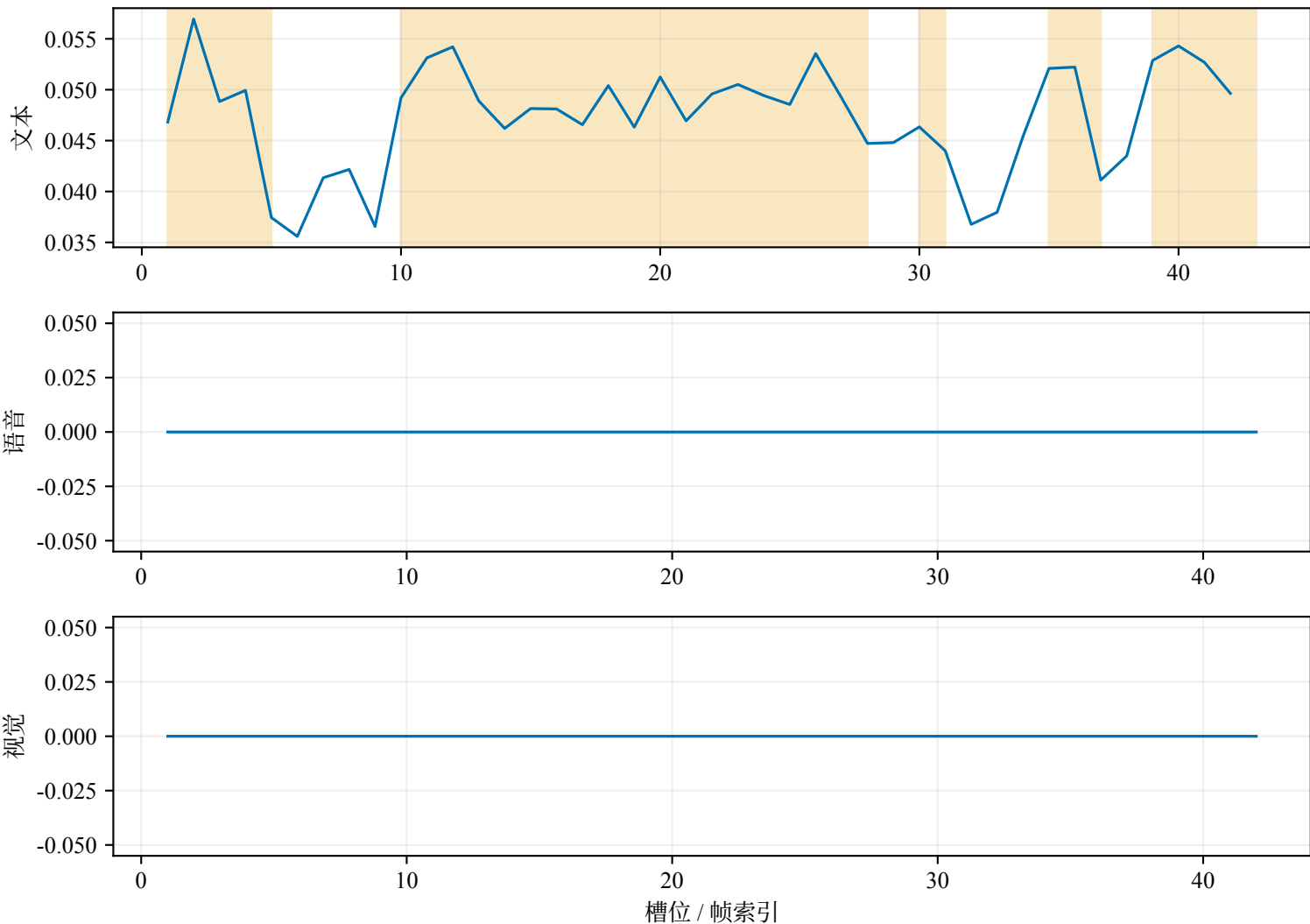
样本 12 正向 Grad×Input (阴影=支持当前预测的关键证据)
