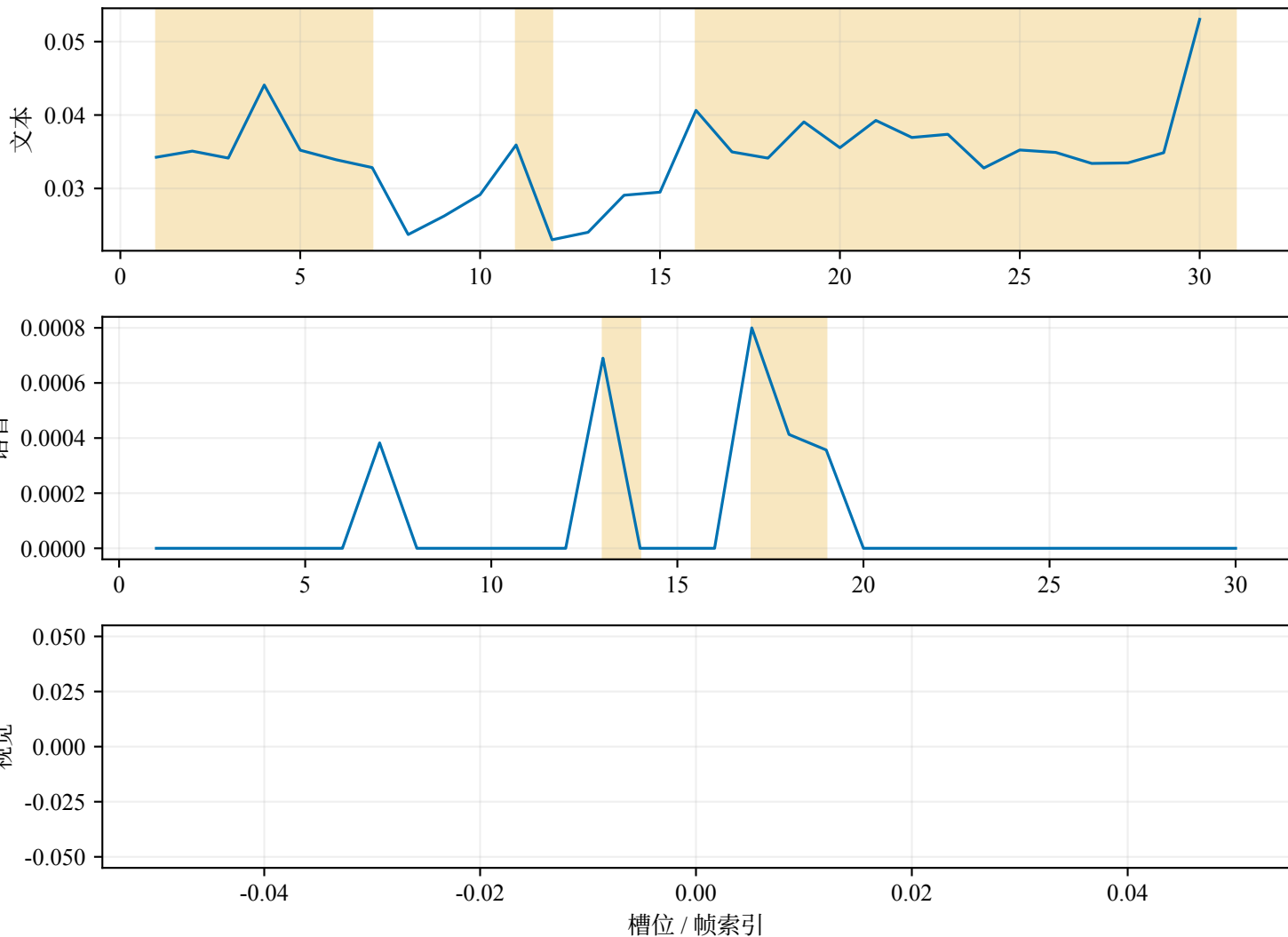
样本 13 正向 Grad×Input (阴影=支持当前预测的关键证据)
