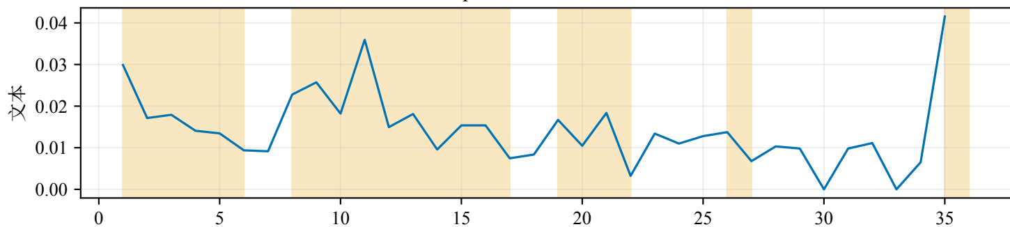
样本 14 正向 Grad×Input (阴影=支持当前预测的关键证据)
