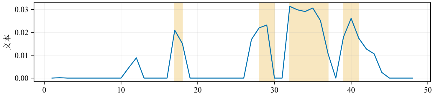
样本 18 正向 Grad×Input (阴影=支持当前预测的关键证据)
