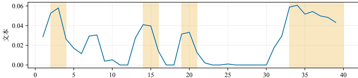
样本 19 正向 Grad×Input (阴影=支持当前预测的关键证据)
