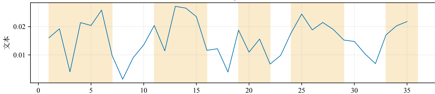
样本 06 正向 Grad×Input（支持当前预测）
