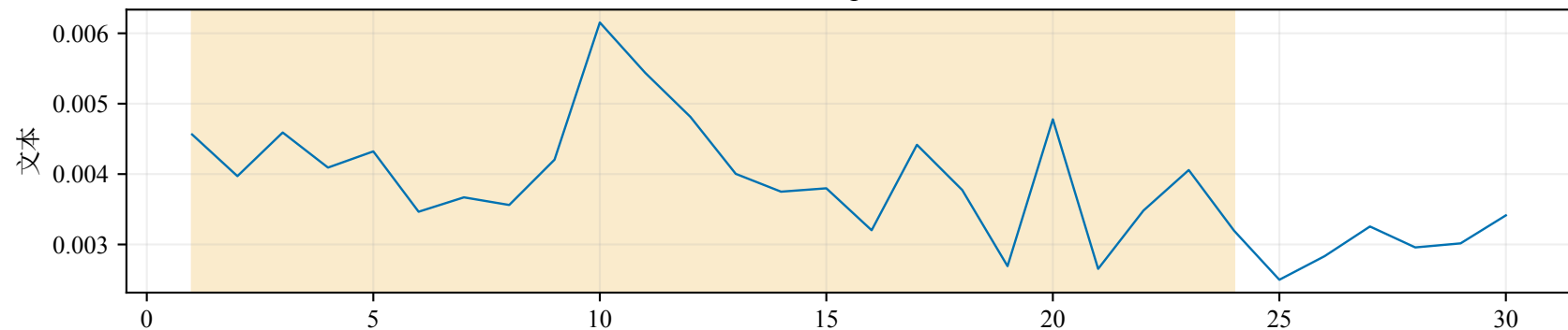
样本 10 正向 Grad×Input (支持当前预测)
